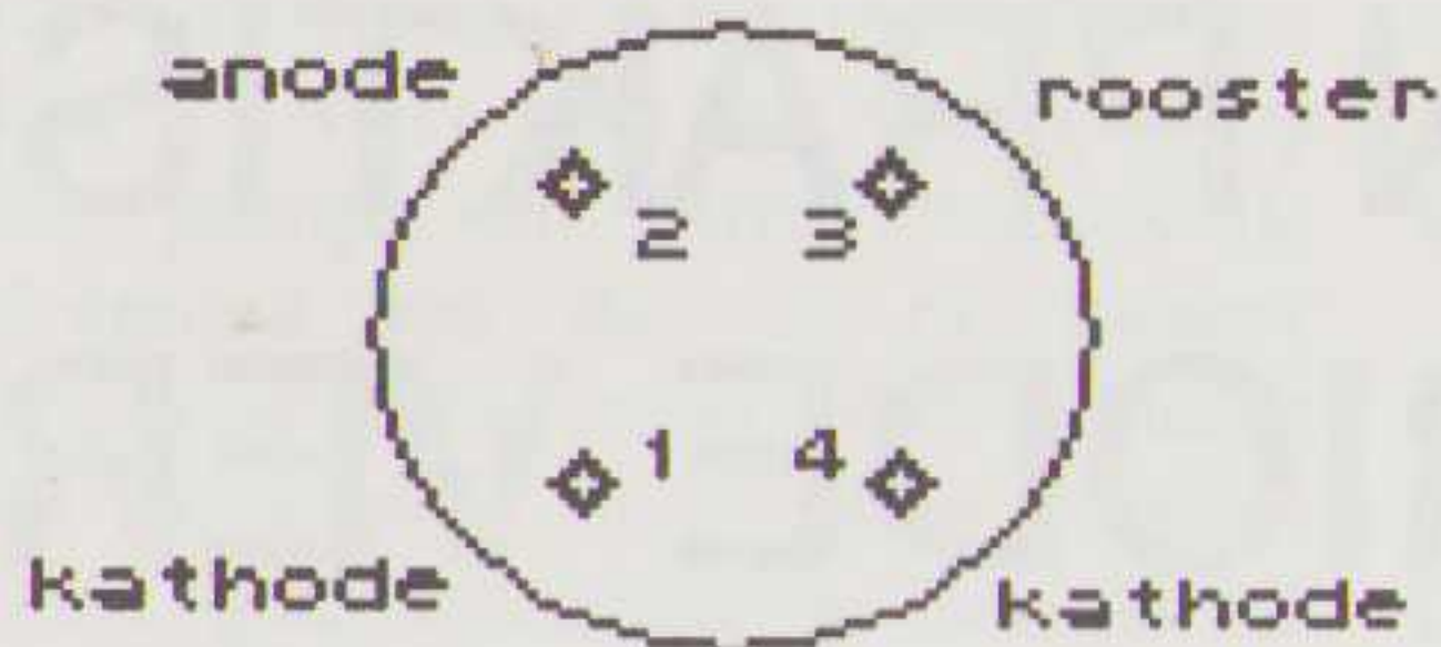
VT25
